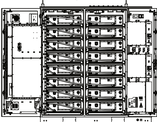
INNENANSICHT/ SYSTEMAUFBAU
